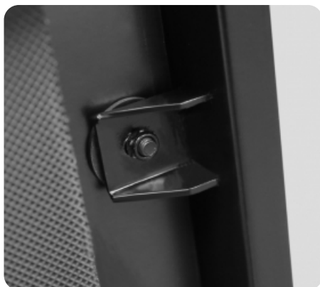
Амортизационная система на основе 8 плоских эластомеров
